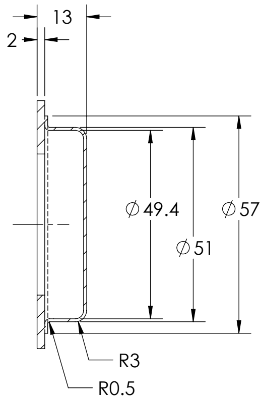
SECTION A-A
